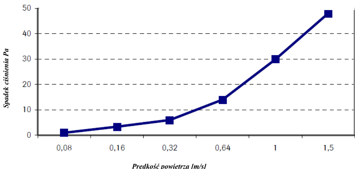
Spadek ciśnienia - w zależności od prędkości przepływu powietrza przez materiał
