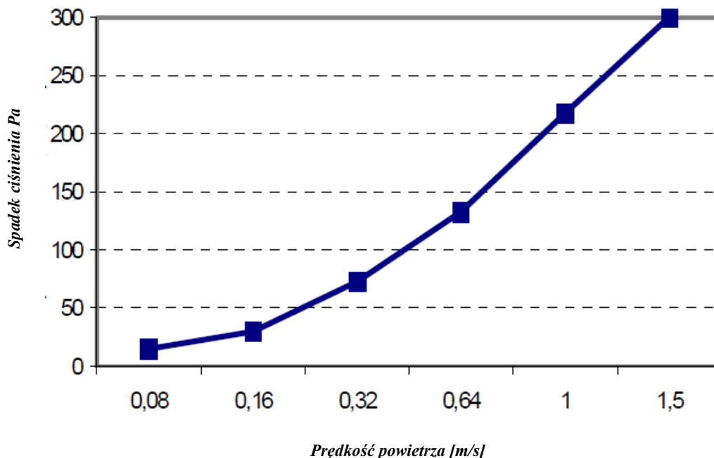
Spadek ciśnienia - w zależności od prędkości przepływu powietrza przez materiał
