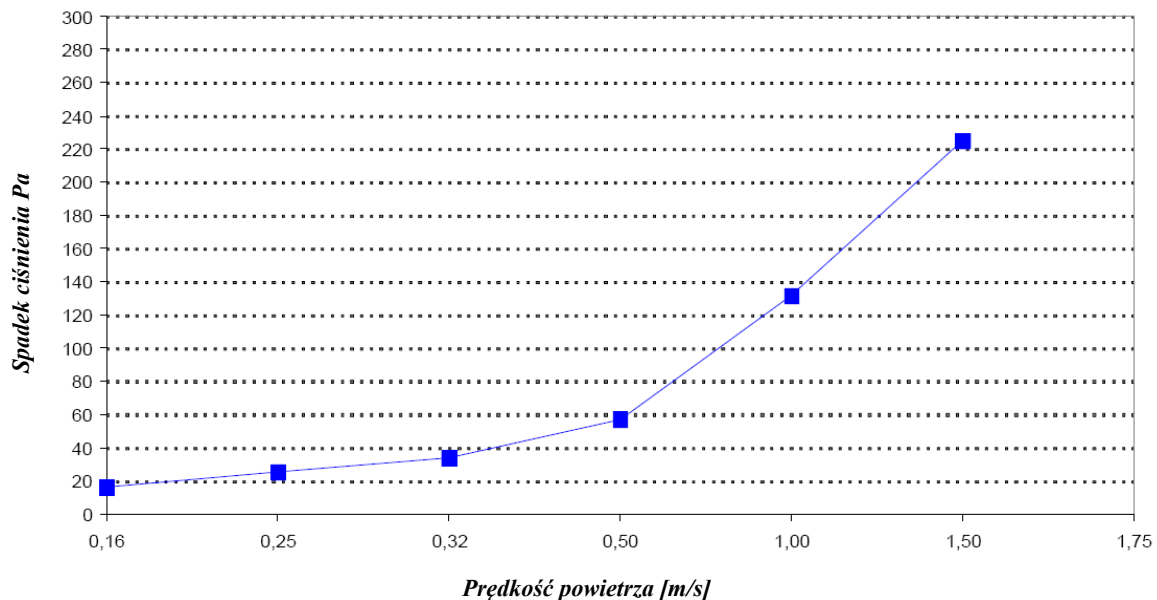
Spadek ciśnienia - w zależności od prędkości przepływu powietrza przez materiał
