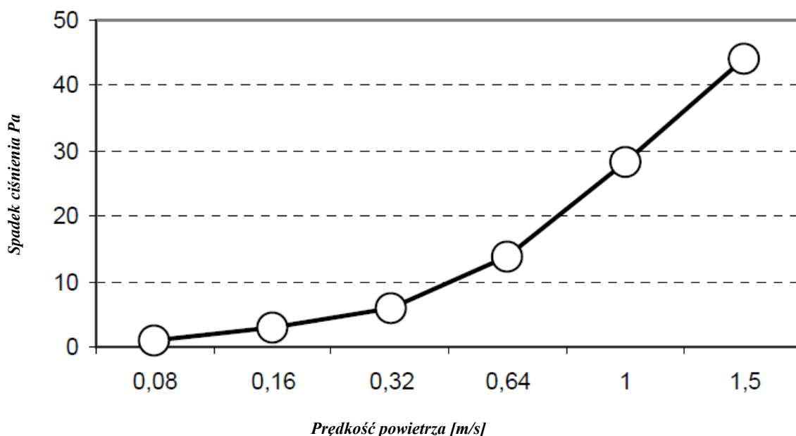
Spadek ciśnienia - w zależności od prędkości przepływu powietrza przez materiał
