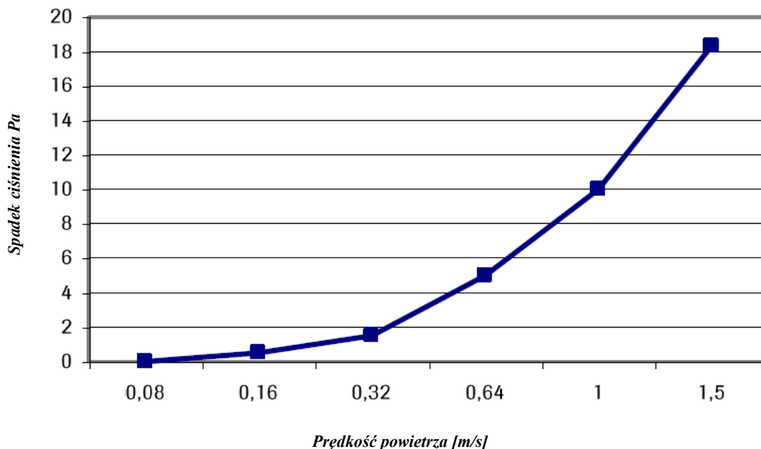
Spadek ciśnienia - w zależności od prędkości przepływu powietrza przez materiał
